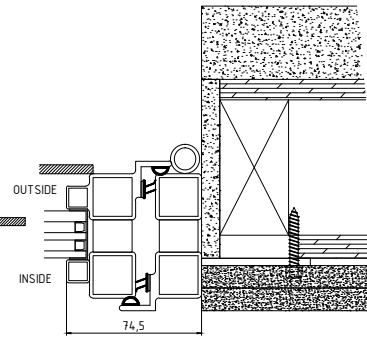
JAMB & STILE
