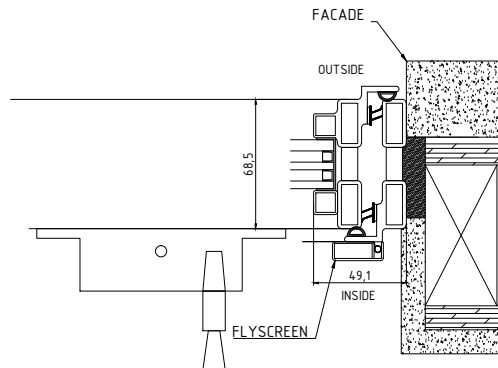
JAMB & STILE
